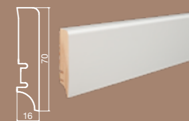
Плинтус для пола Белый окрашенный PW70 – P7027362A
