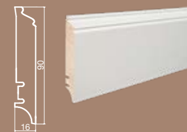
Плинтус для пола Белая пленка P90 – P9027362A
