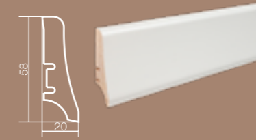
Плинтус для пола Белая пленка P20 – P2018101A
