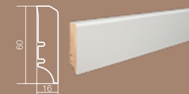
Плинтус для пола Белая пленка P90 – P9027362A
